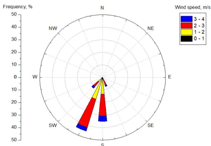
2 paveikslas. Vėjo greitis ir kryptys
