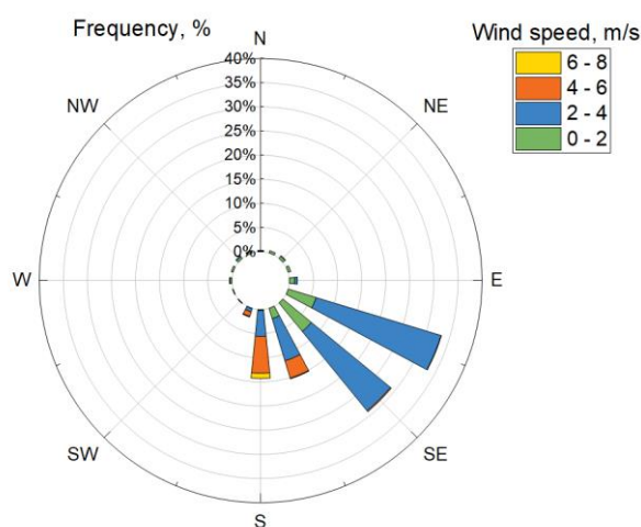
2 Pav. Vėjo kryptys ir greitis
